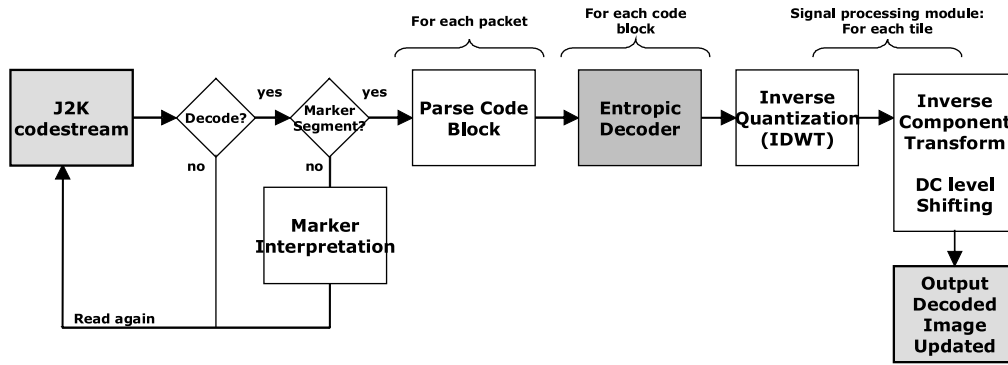
Fig. 15. Decoder synopsis.
