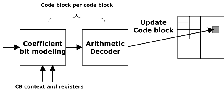
Fig. 16. Entropic decoder.
